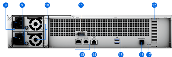
Задняя панель
