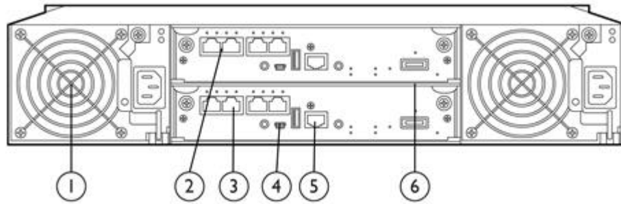
P2000 G3 iSCSI dual controller
